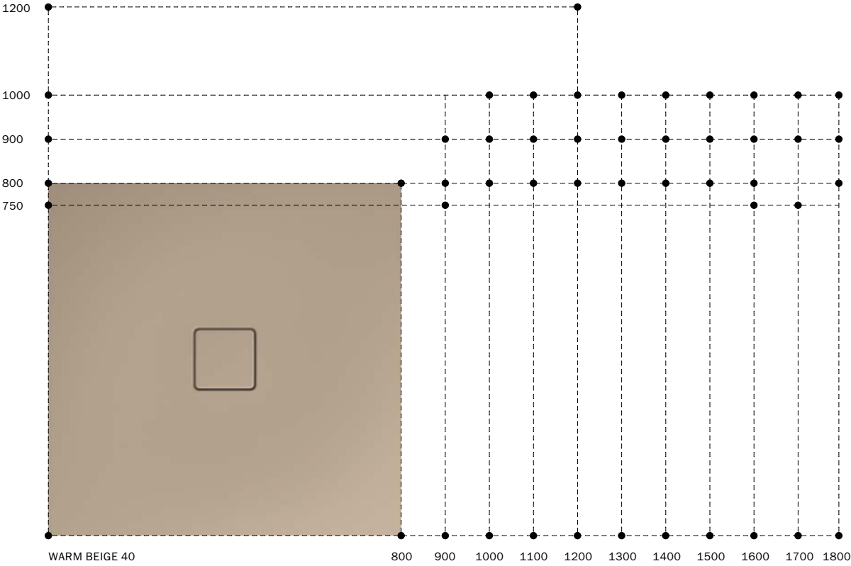
CONOFLAT (S. 22)
