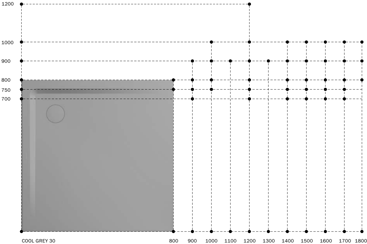
SUPERPLAN (S. 24)
